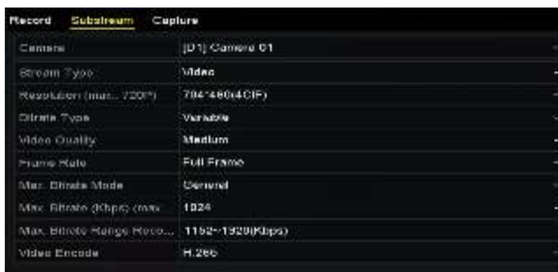
Рисунок 5-5 Параметры доп. потока
