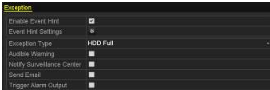
Рисунок 8-13 Меню настройки исключений
