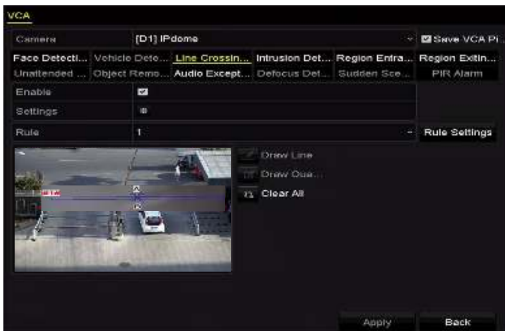
Рисунок 10-6 Нарисуйте линию для обнаружения пересечения линии
