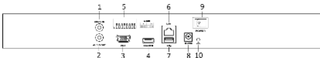
Рисунок 1-12 Серии DS-7600NI-I2 и DS-7600NI-K2
