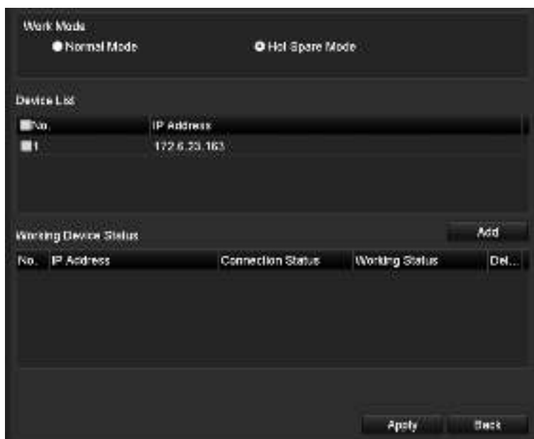
Рисунок 7-16 Добавление рабочих устройств
