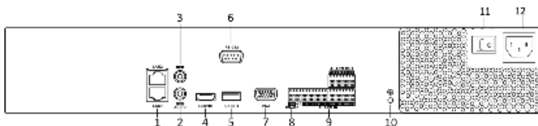
Рисунок 1-16 Серии DS-7700NI-I4 и DS-7700NI-K4
