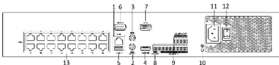
Рисунок 1-17 Серии DS-7700NI-I4/16P и DS-7700NI-K4/16P
