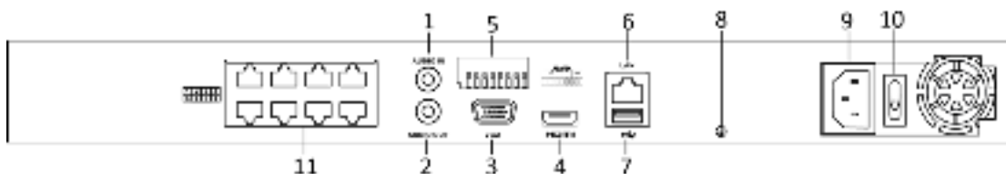
Рисунок 1-13 Серии DS-7600NI-I2/8P и DS-7600NI-K2/8P
