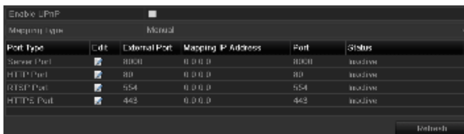
Рисунок 12-22 Меню настройки UPnP™
