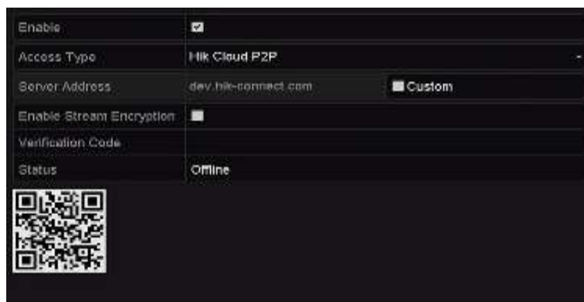
Рисунок 12-2 Меню настройки Hik Cloud P2P
