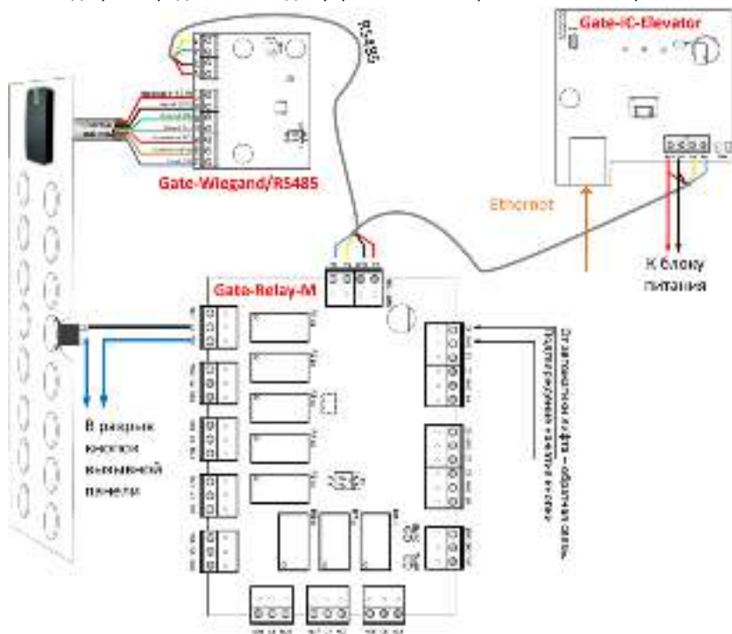
Рис.2. Схема подключения
