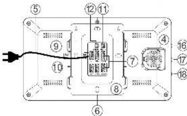
Конструкция монитора
