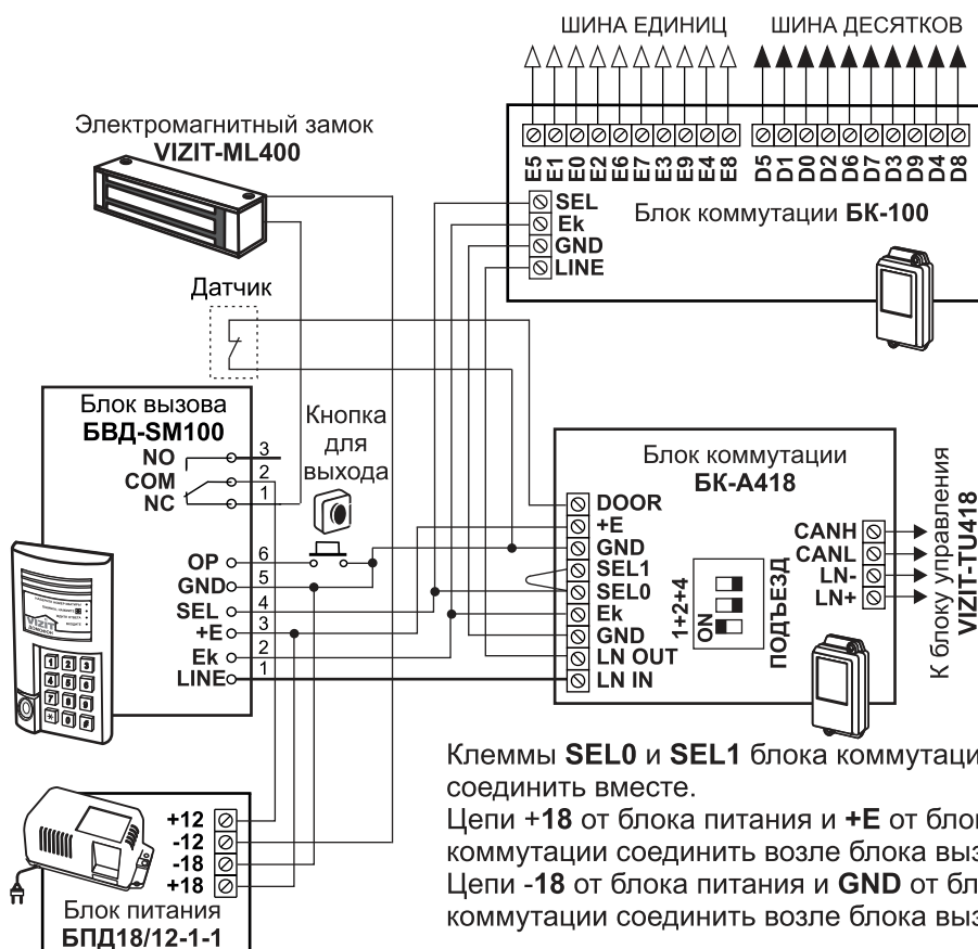
Рисунок 1 - Пример включения блока коммутации в составе 100-квартирного домофона с блоком вызова БВД-СМ100
