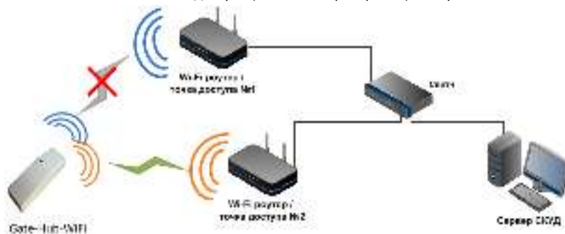
Рис 5. Работа с несколькими Wi-Fi точками доступа
