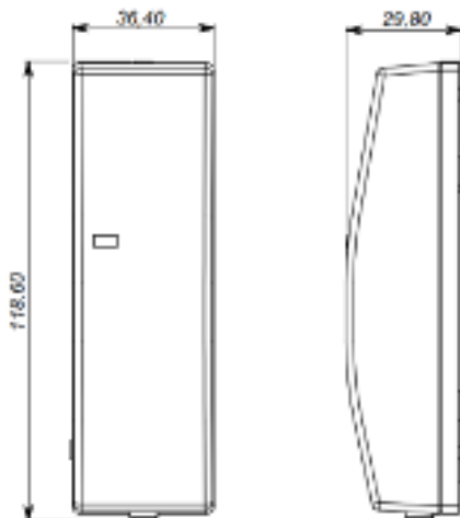
Рис 8. Габаритные размеры
