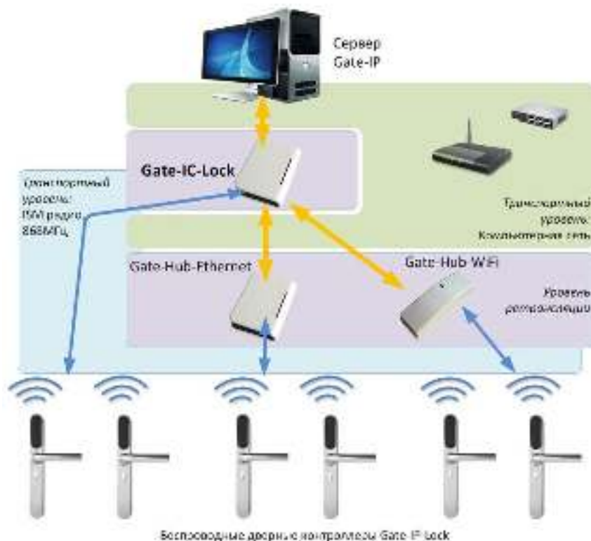
Рис 6. Построение системы беспроводных замков
