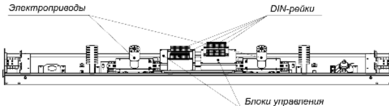
Рисунок 3. Вид балки привода турникета PERCo-RTD-20.1 без крышки
