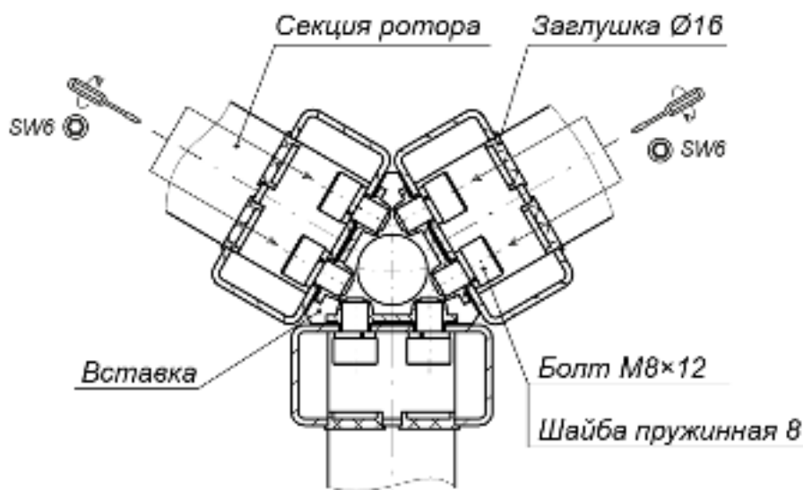
Рисунок 19. Схема соединения секций ротора
