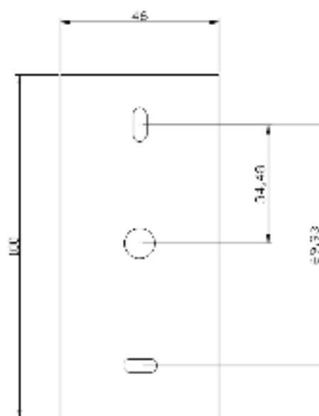
Монтажный чертёж
