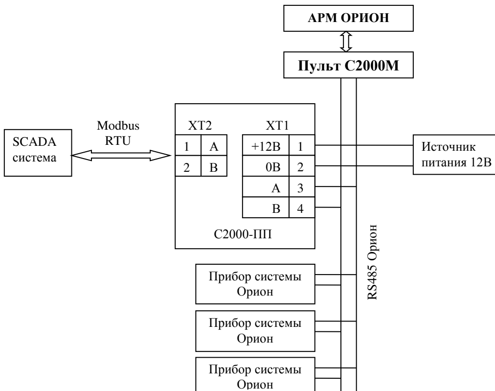
Рисунок 17. Подключение «С2000-ПП» в режиме «Орион-Slave»
