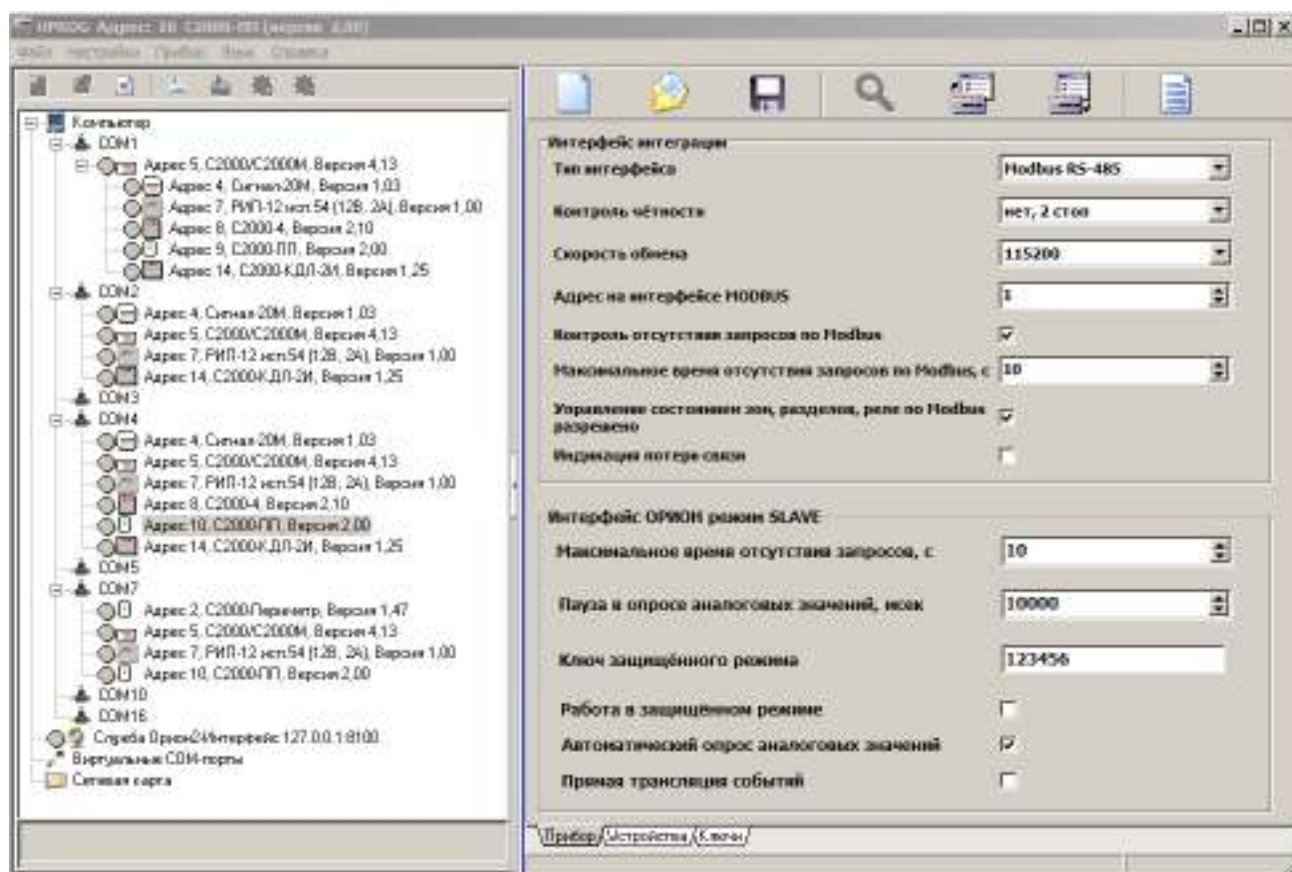
Рисунок 6. Конфигурационные параметры. Страница «Прибор»
