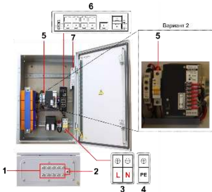
Рис. 3 Подключение уличного коммутатора на примере OS-46TB1(SW-60812/I)
