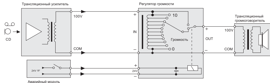
Схема подключения
