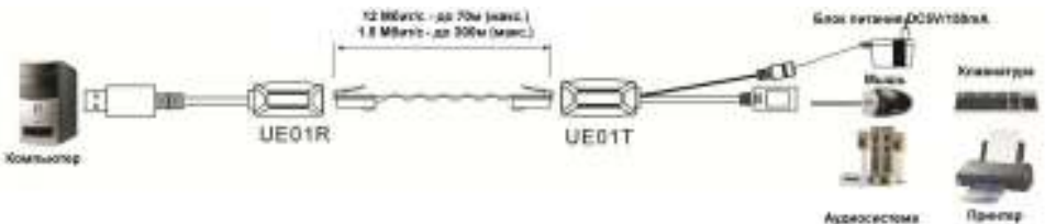
Рис. 5 Схема подключения передатчика UE01T и приёмника UE01R.
