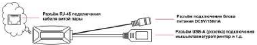
Рис.3 Разъёмы передатчика UE01T
