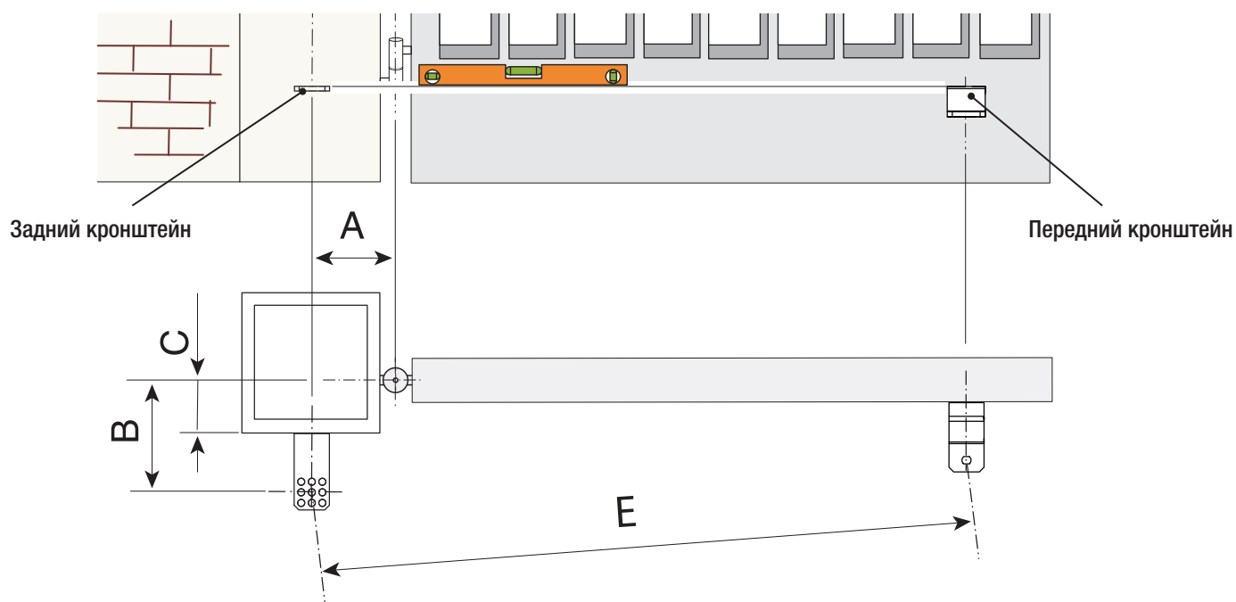
Установочные размеры (мм)
