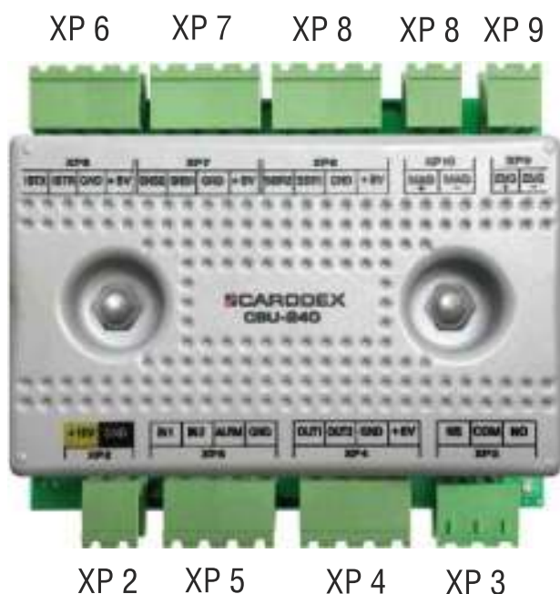
Рисунок 6.3.1 Контроллер управления турникетом «CBU-240»
