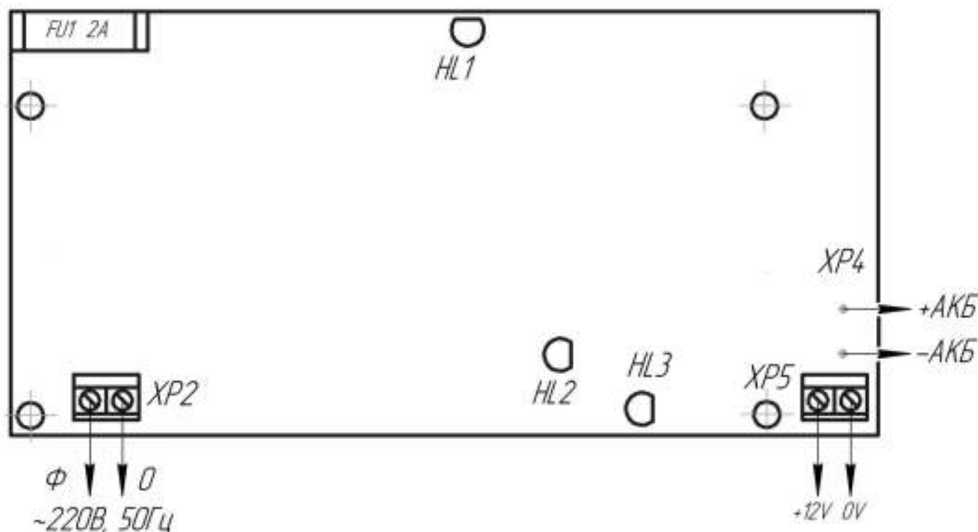
Рис. 1 Схема подключения
