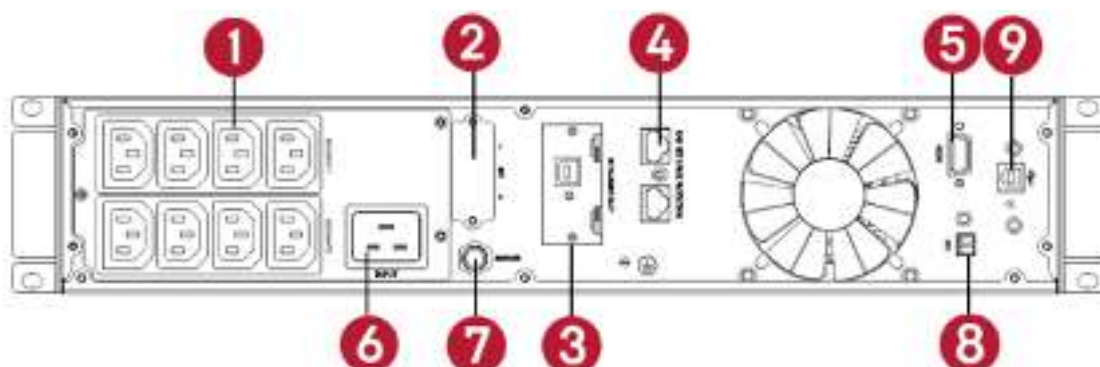
Рисунок 2-1. Вид задней панели ИБП 1 кВ·А и 1,5 кВ·А
