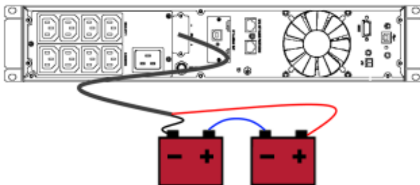
Рисунок 2-13. Подключение внешних аккумуляторных батарей
