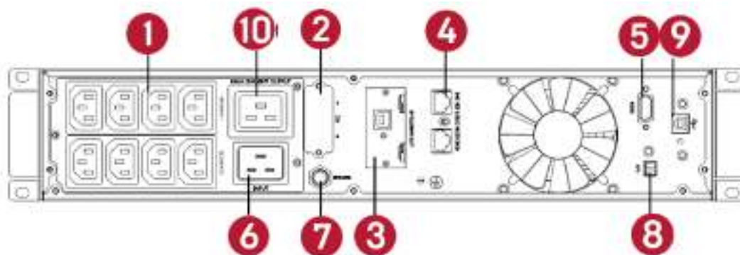
Рисунок 2-3. Вид задней панели ИБП 3 кВ·А
