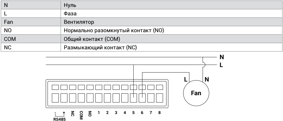
Рис. 2.2 Схема подключения интерфейса переменного тока.
