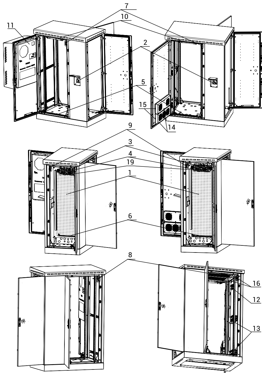
Рисунок 7. Общий вид шкафов серии ШТБ-2
