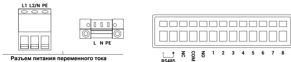
Рис. 2.1 Интерфейс подключения (данные о порте энергопровода содержатся в указаниях на заводской табличке с паспортными данными)
