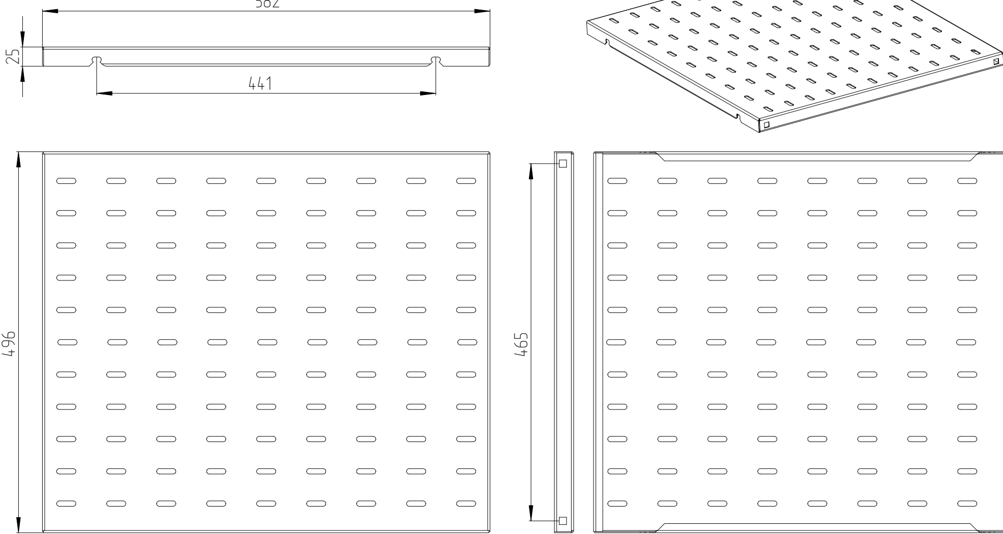
ПОЛКА СВ-58У
