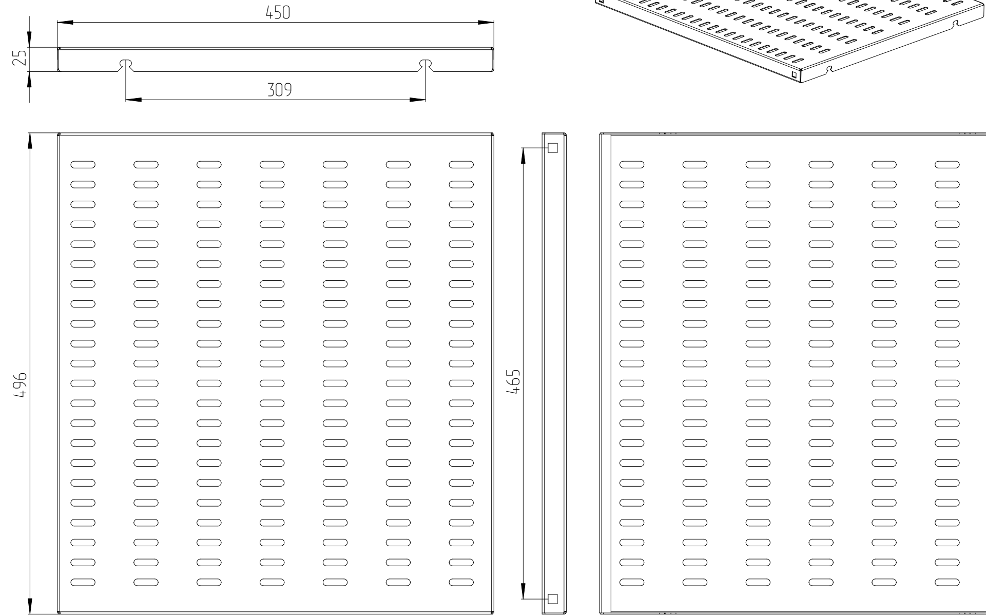
ПОЛКА СВ-58
