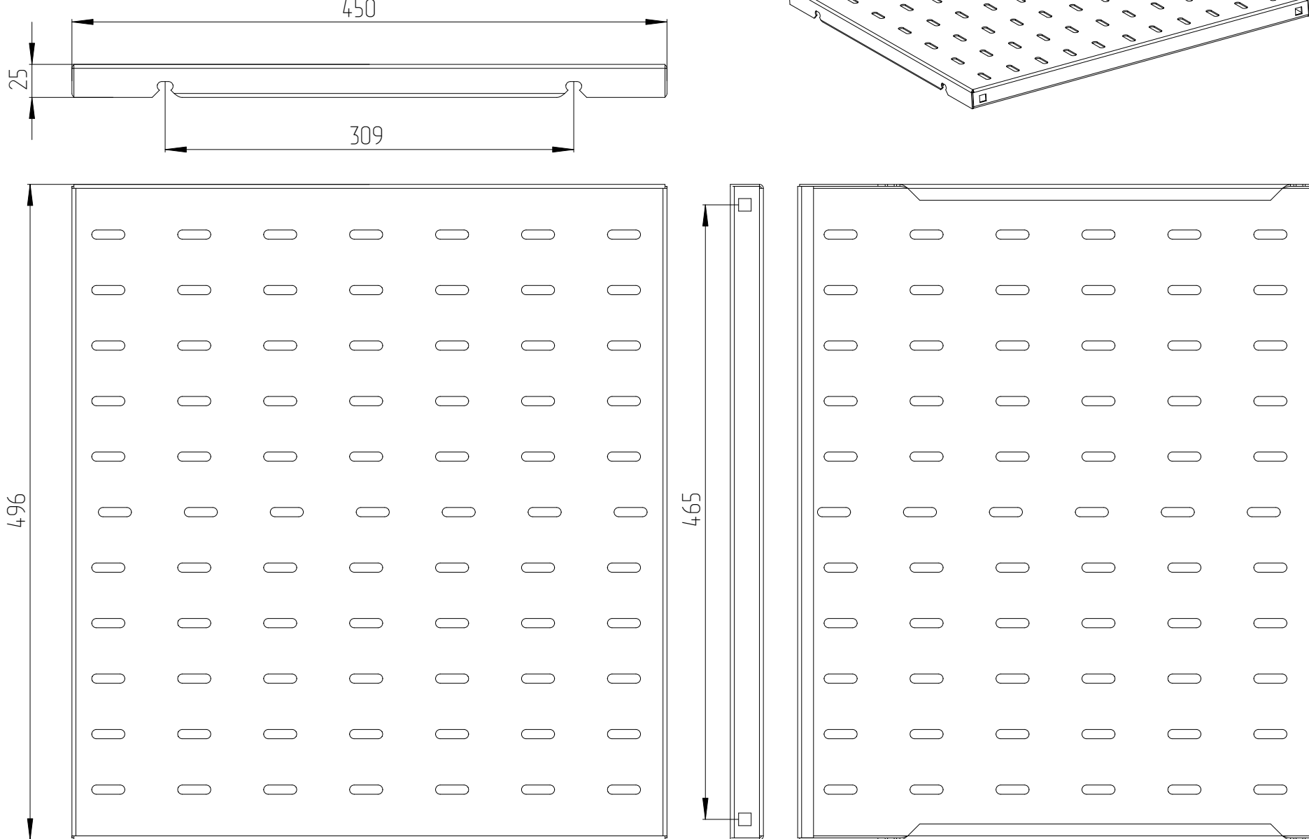
ПОЛКА СВ-58У
