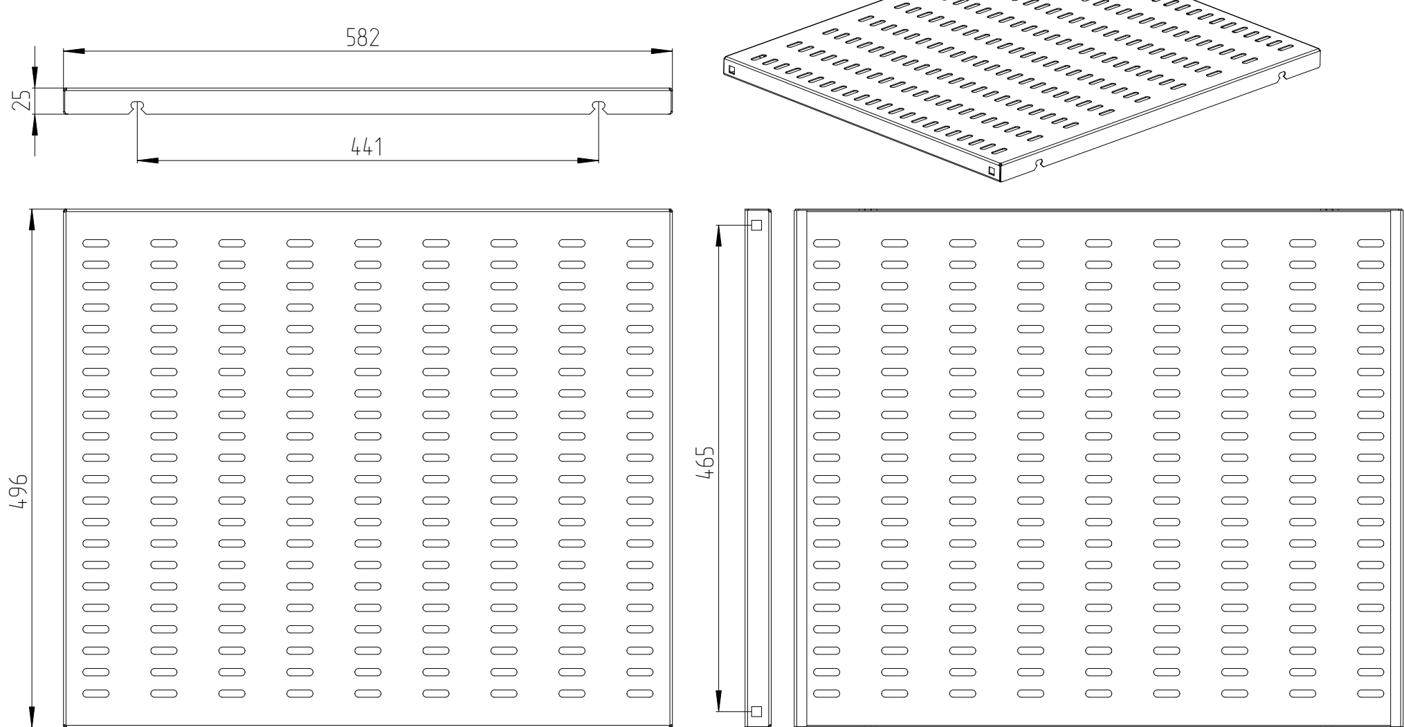
ПОЛКА СВ-58
