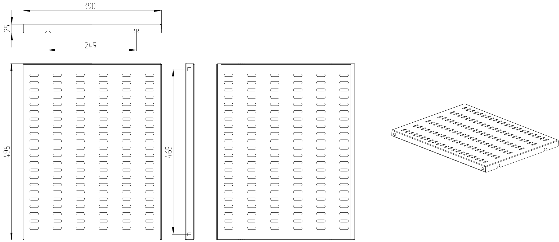
ПОЛКА СВ-45
