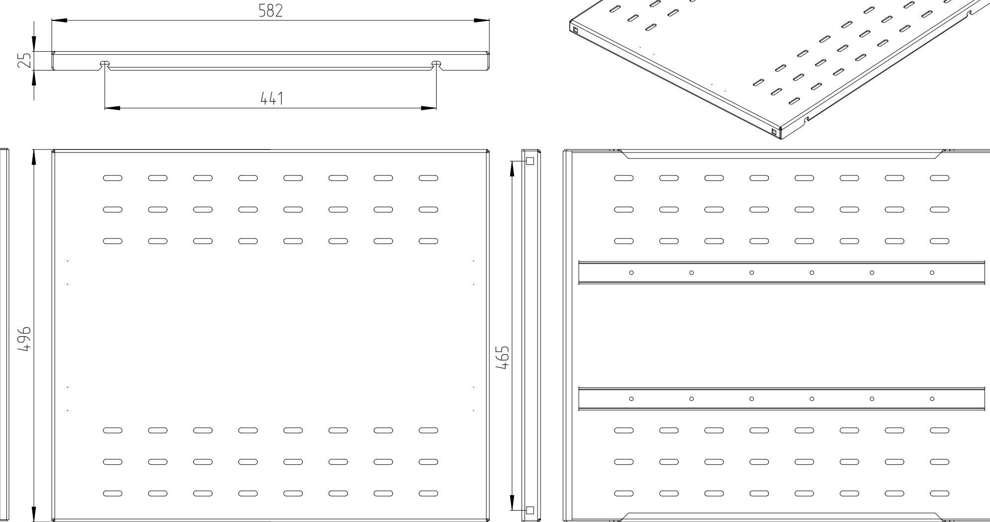
ПОЛКА СВ-58АК
