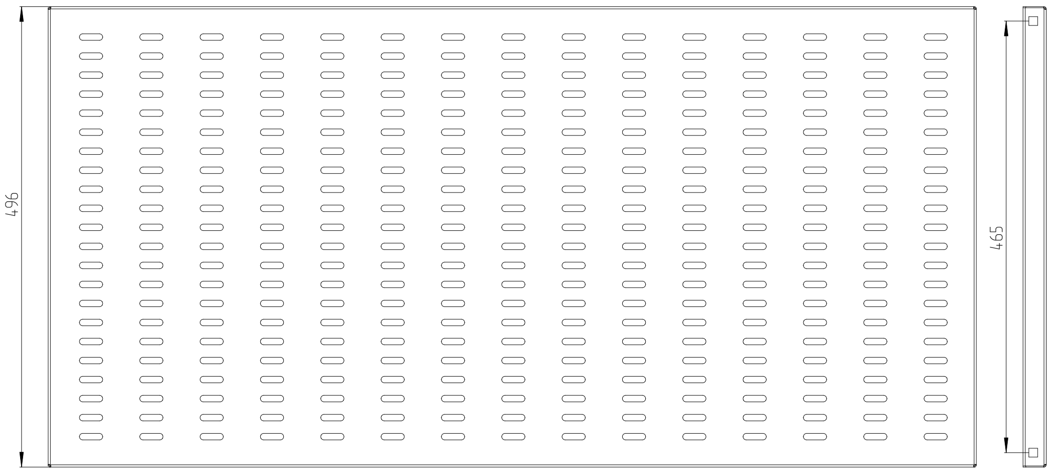
ПОЛКА СВ-100У
