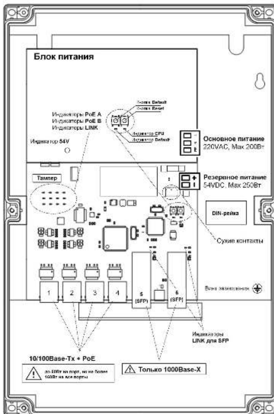
Рисунок 3.2 - Расположение элементов коммутатора PSW-2G+
