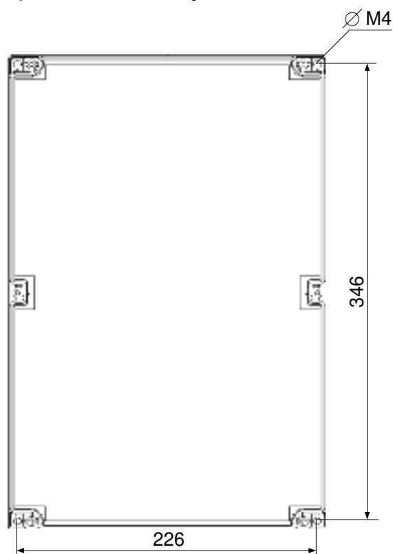
Рисунок 7.1 - Разметка крепления
