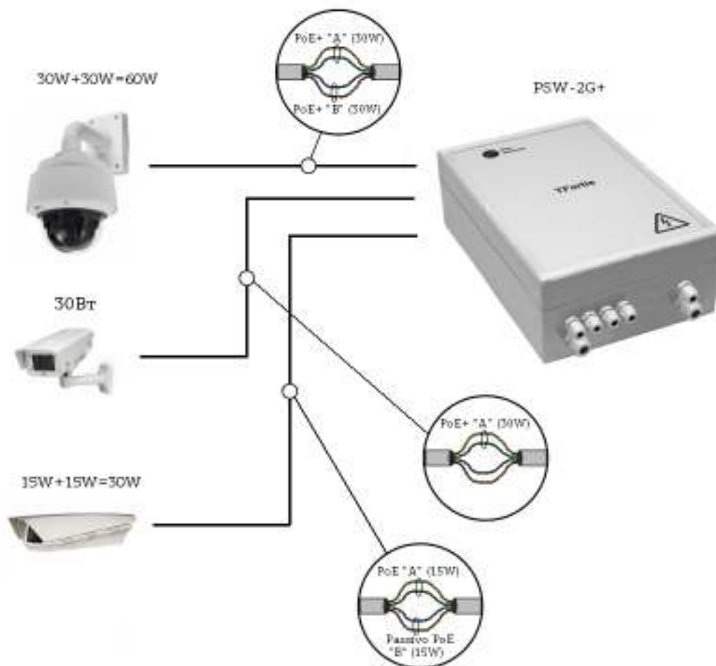
Рисунок 3.3 - Схема питания по PoE для разных случаев
