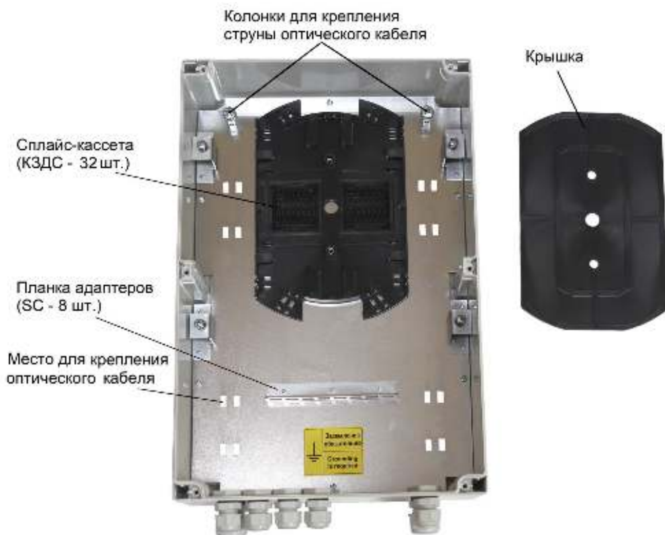
Рисунок 3.4 - Оптический кросс
