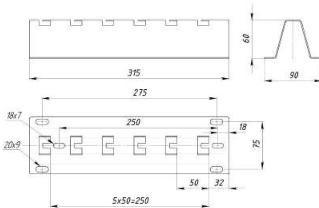
Рисунок 2 – Конструктивное исполнение кронштейна универсального быстрой фиксации EWT-UWB-300-1,5-SZ
