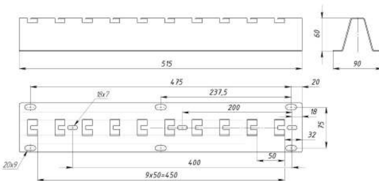
Рисунок 2 – Конструктивное исполнение кронштейна универсального быстрой фиксации EWT-UWB-500-1,5-SZ
