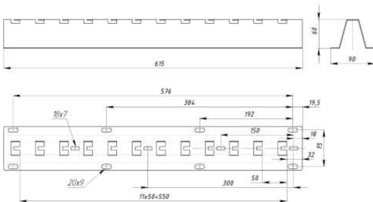
Рисунок 2 – Конструктивное исполнение кронштейна универсальной быстрой фиксации EWT-UWB-600-1,5-SZ
