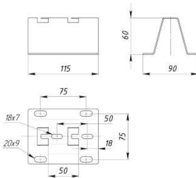
Рисунок 1 – Конструктивное исполнение кронштейна универсального быстрой фиксации EWT-UWB-100-1,5-SZ
