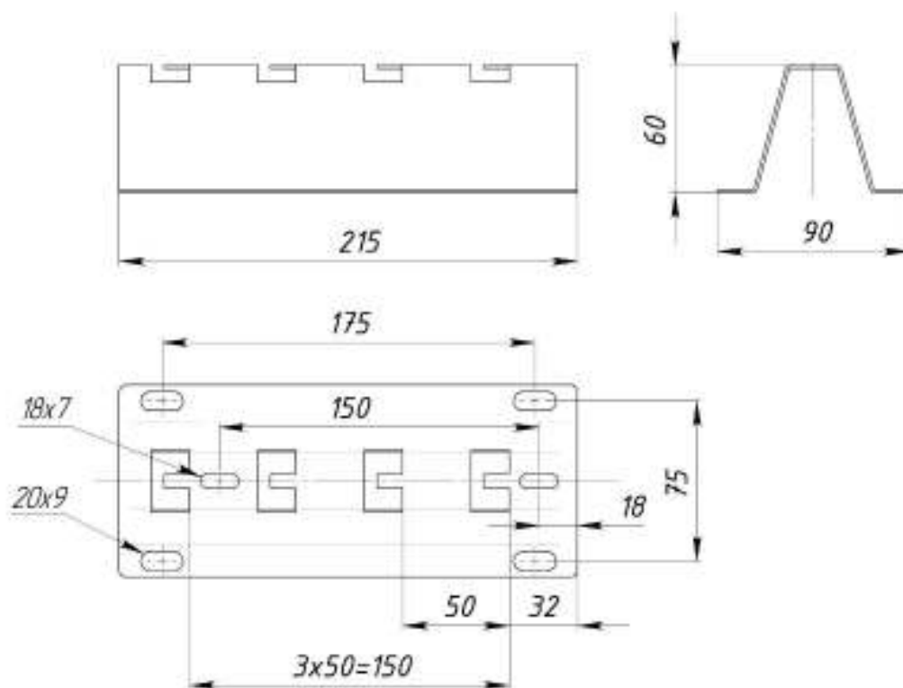
Рисунок 2 – Конструктивное исполнение кронштейна универсального быстрой фиксации EWT-UWB-200-1,5-SZ
