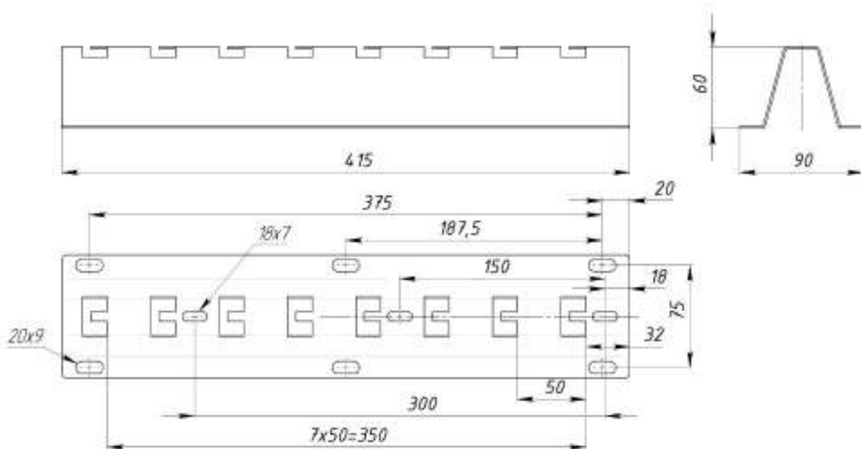
Рисунок 2 – Конструктивное исполнение кронштейна универсального быстрой фиксации EWT-UWB-400-1,5-SZ
