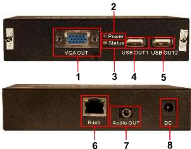
Рис. 3 Приемник RLN-VKM/1, разъемы и индикаторы на передней и задней панелях
