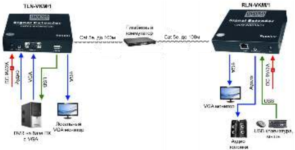
Рис. 5 Схема подключения комплекта TLN-VKM/1+RLN-VKM/1 в режиме «точка-точка» через гигабитный коммутатор
