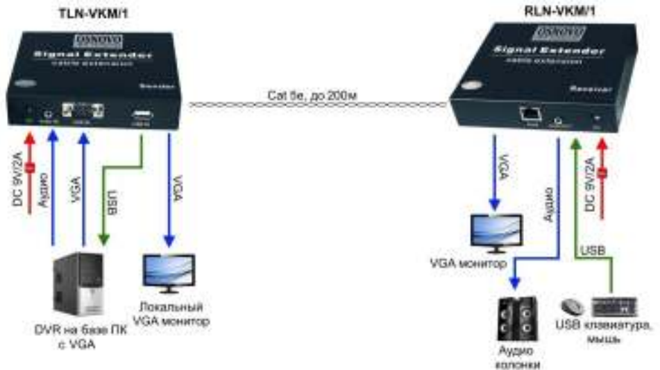
Рис.4 Схема подключения комплекта TLN-VKM/1+RLN-VKM/1 в режиме «точка-точка»
