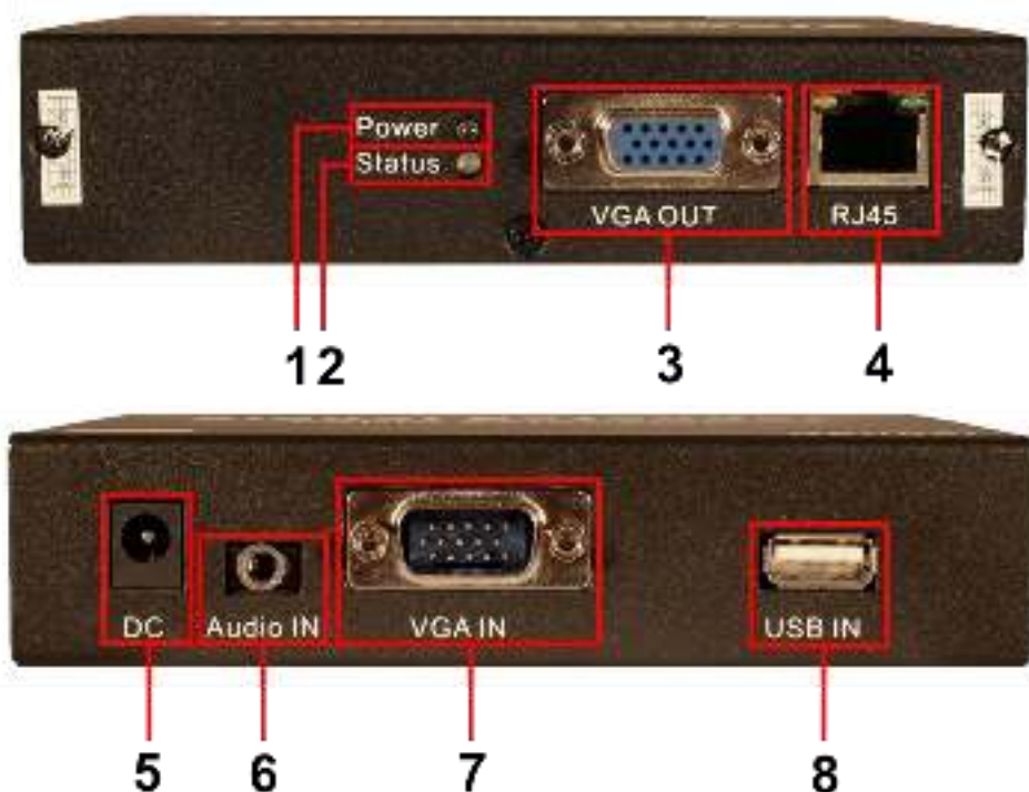
Рис. 2 Передатчик TLN-VKM/1, разъемы и индикаторы на передней панели
