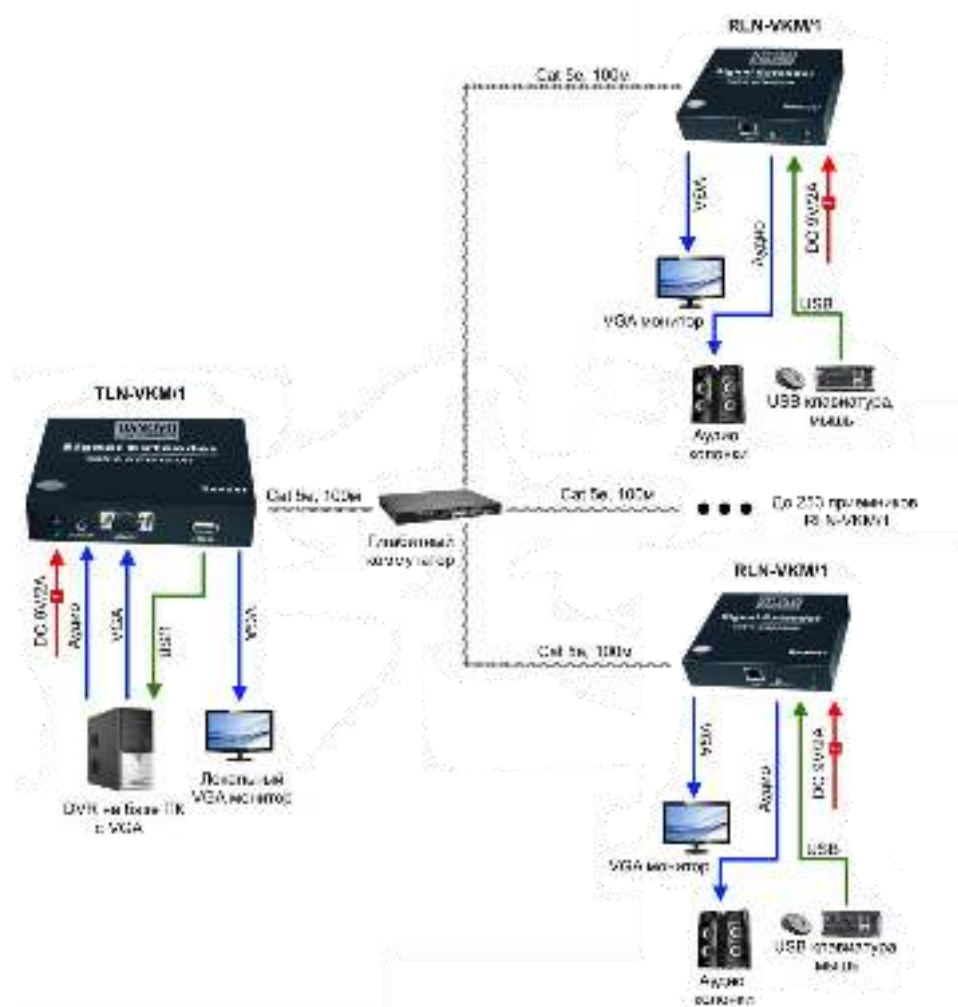
Рис. 6 Схема подключения комплекта TLN-VKM/1+RLN-VKM/1 через гигабитный коммутатор в режиме «точка-многоточка»
