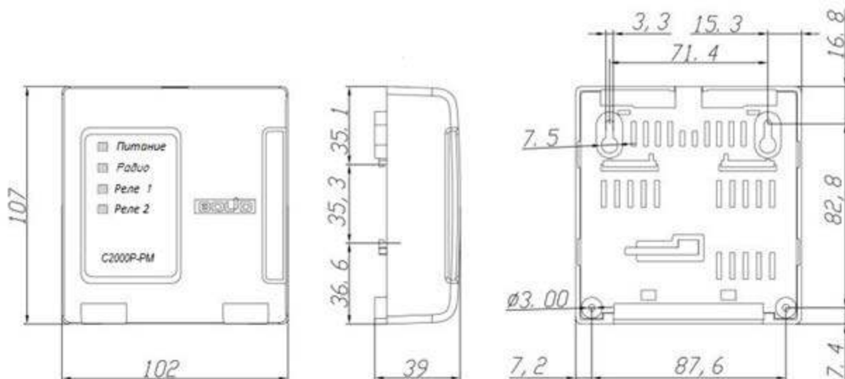
Рисунок 2.3 Монтажные размеры
