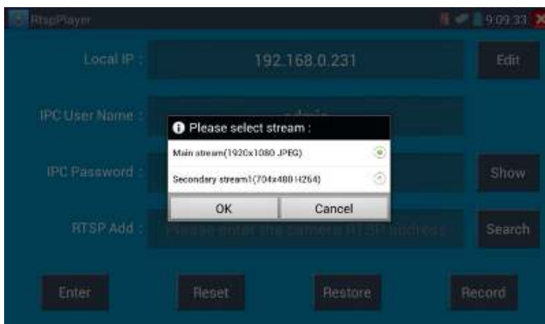
Рис.13 Функция RSTP-результат
