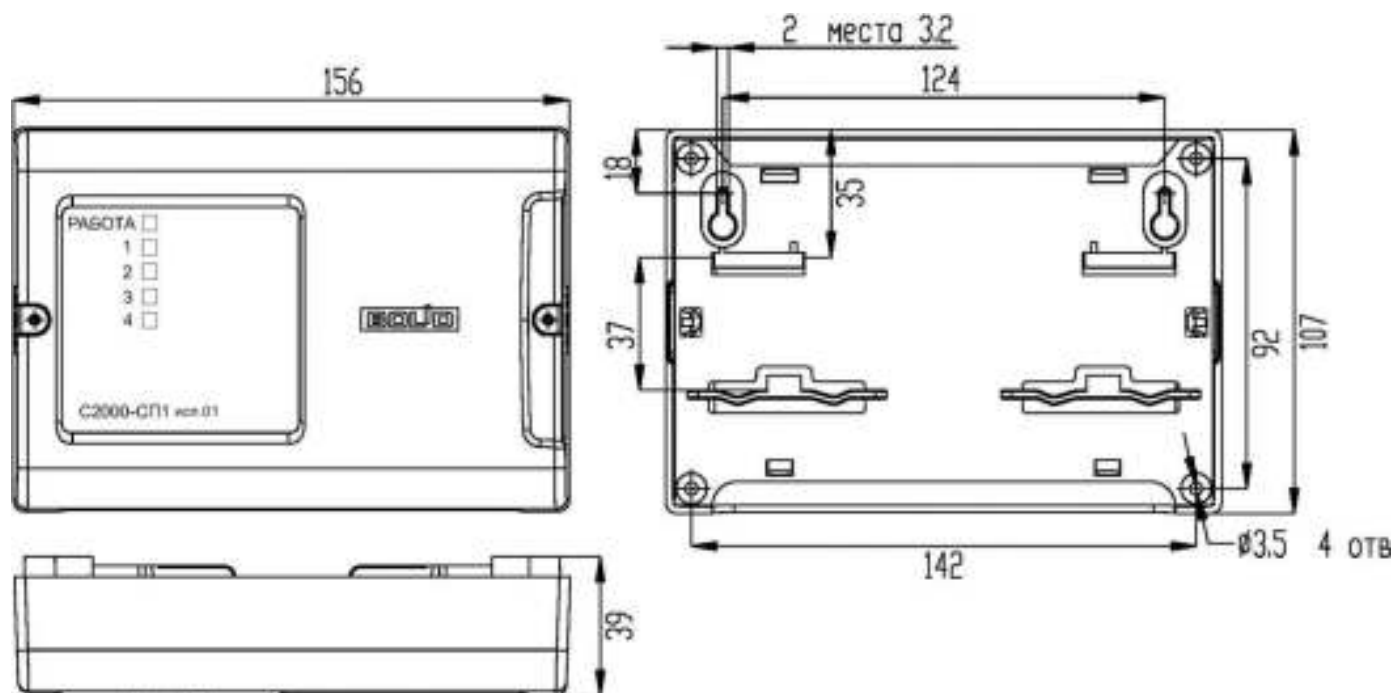
Рисунок 2.2.2.2. Габаритные и установочные размеры блока.
