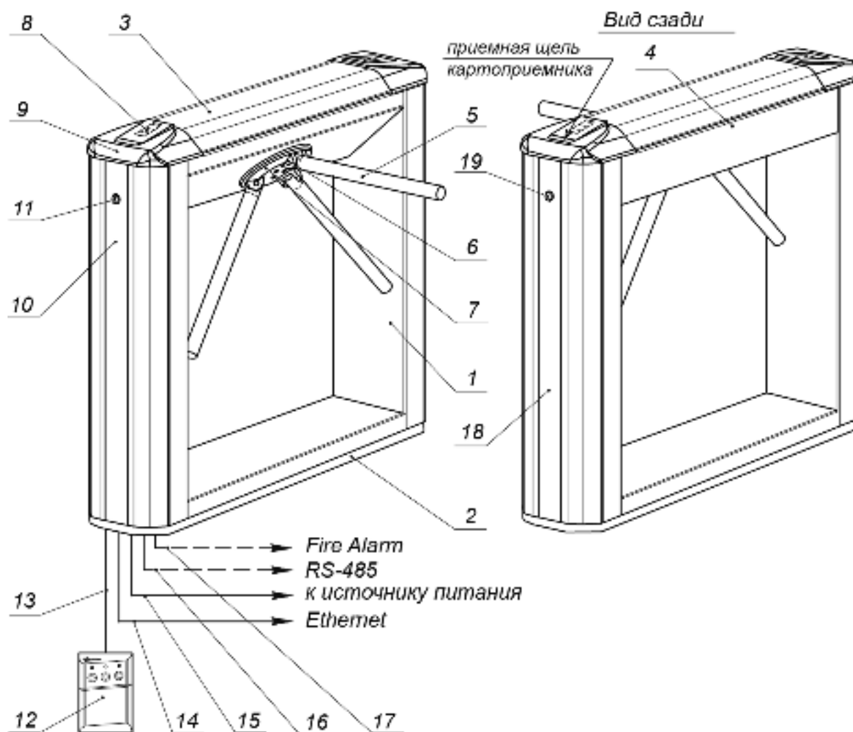
Рисунок 1. Устройство ЭП
