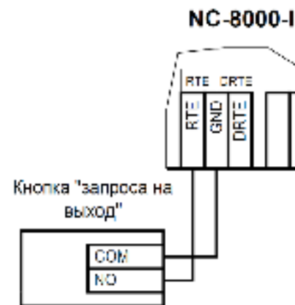
Рисунок 16. Схема подключения кнопки запроса на выход
