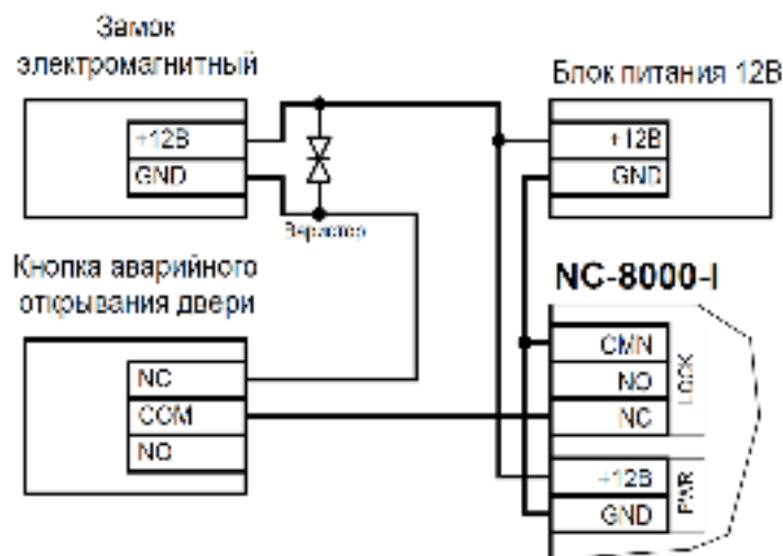
Рисунок 10. Схема подключения замка, запираемого напряжением
