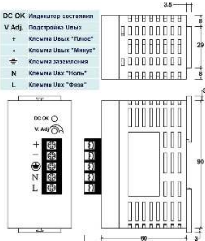
Габаритные размеры AD1048FS и обозначения на передней панели
