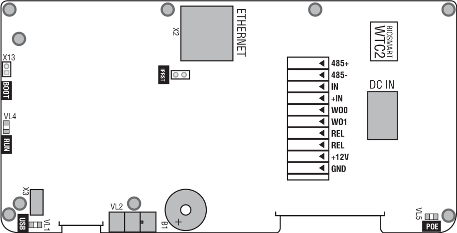
Рисунок 2. Внешний вид печатной платы терминала
