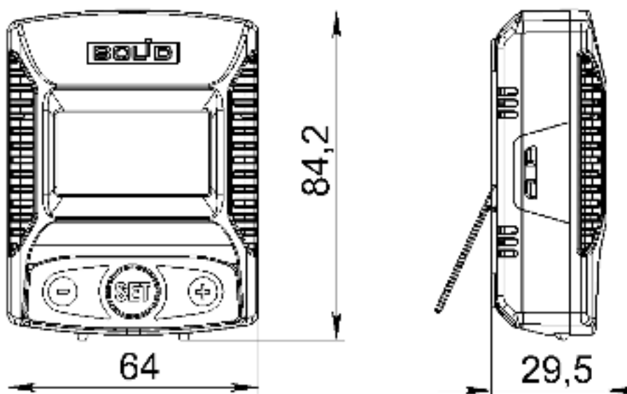
Рис.2.1 Внешний вид и габаритные размеры измерителя «С2000-ВТИ»
