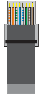
EIA/TIA 568B
