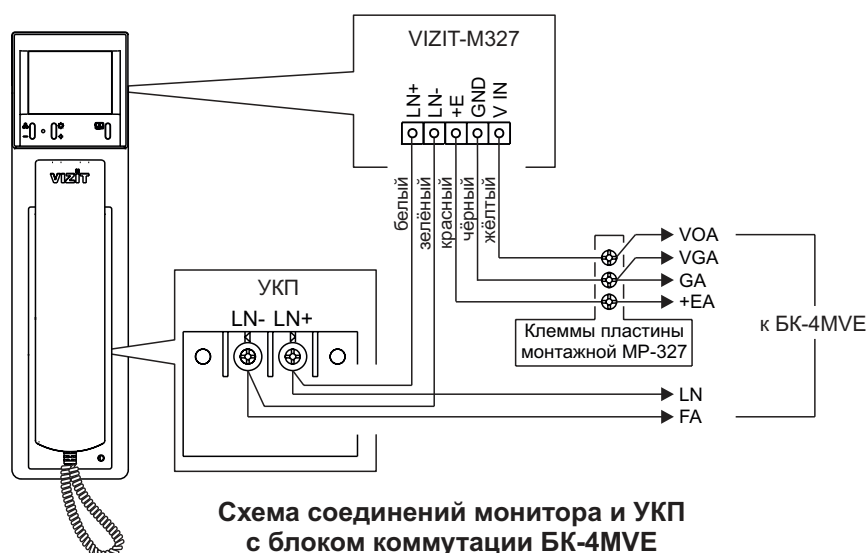
Схема соединений монитора и УКП с блоком коммутации БК-100М и разветвителем сигнала РВЕ-4
