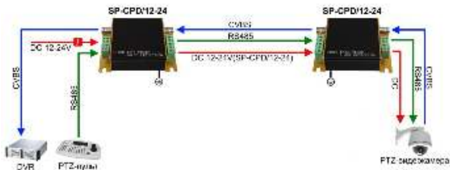
Рис. 3 Подключение SP-CPD/12-24
