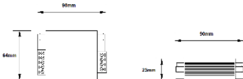
Рис. 2 Габаритные размеры SP-CPD/12-24
