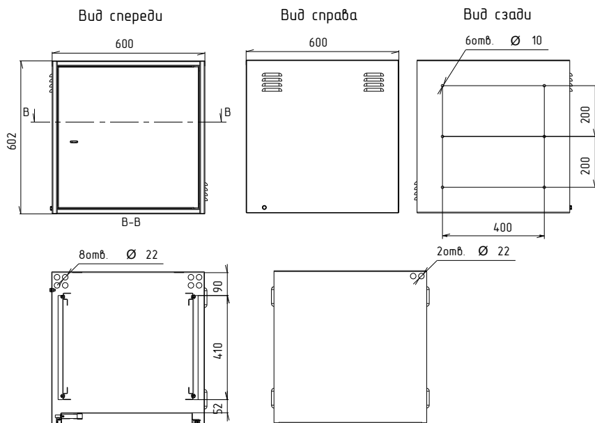
Чертеж шкафа
