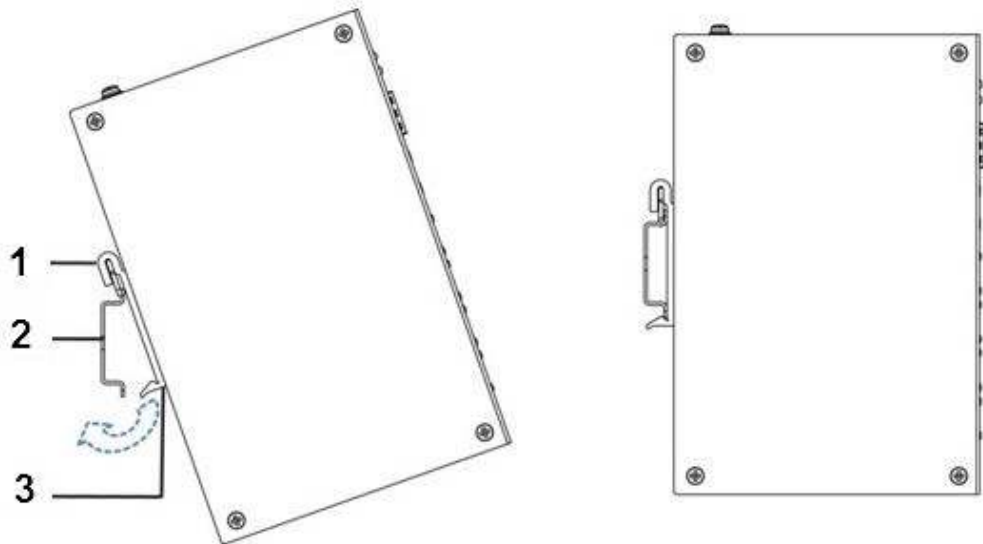
Figure 3-1 DIN rail
