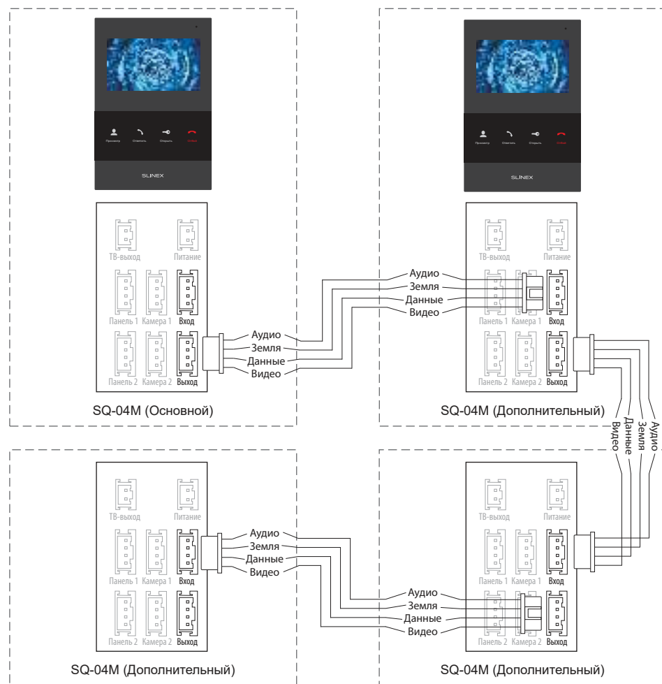
Схема 2. Подключение системы домофонов SQ-04M.
