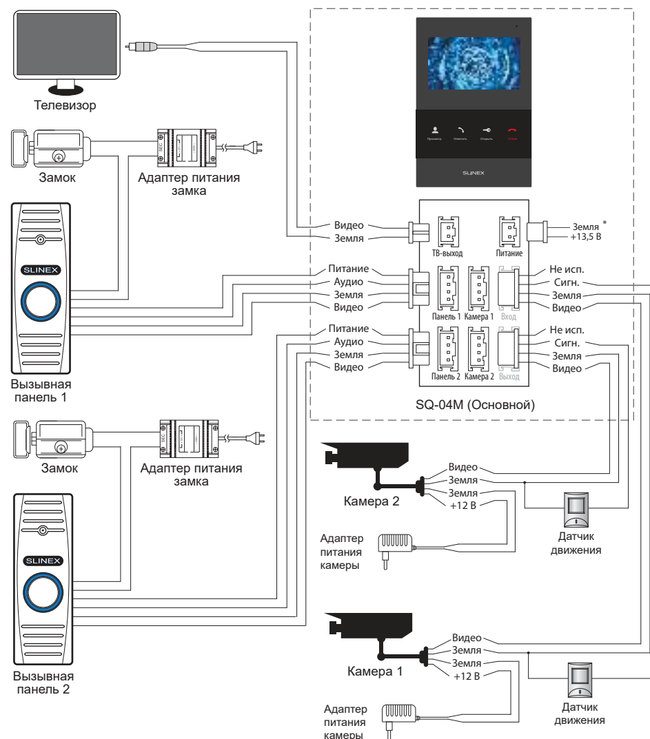
Схема 1. Подключение вызывных панелей, камер и телевизора к домофону SQ-04M
