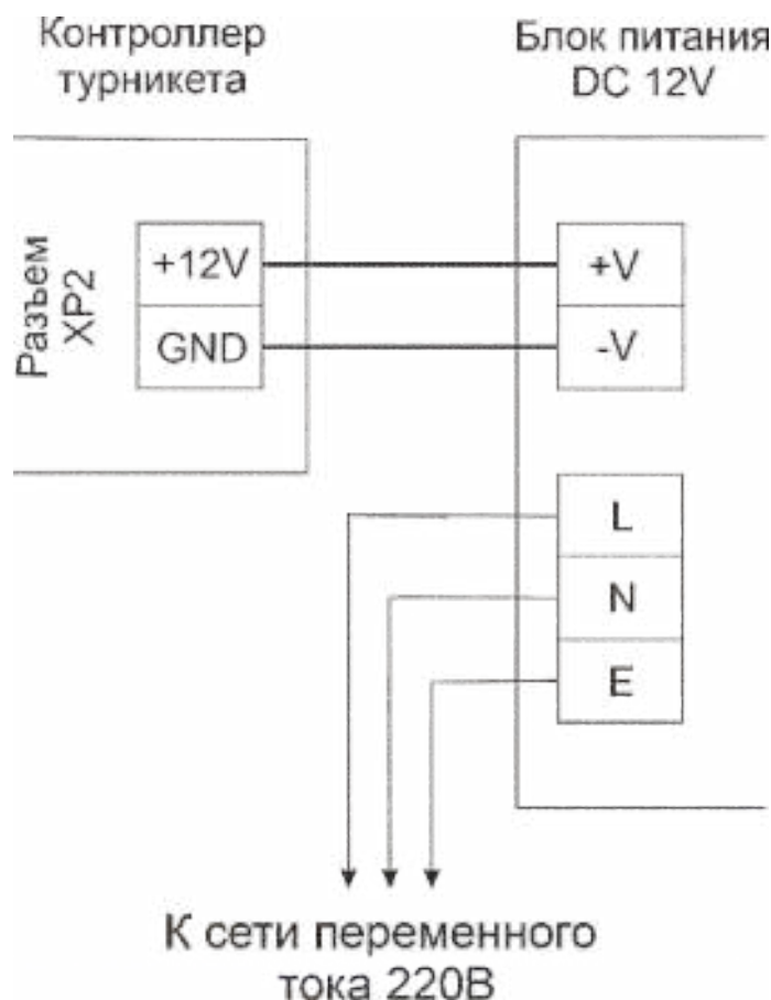
Рисунок 8.4.1 Подключение питания к турникету
