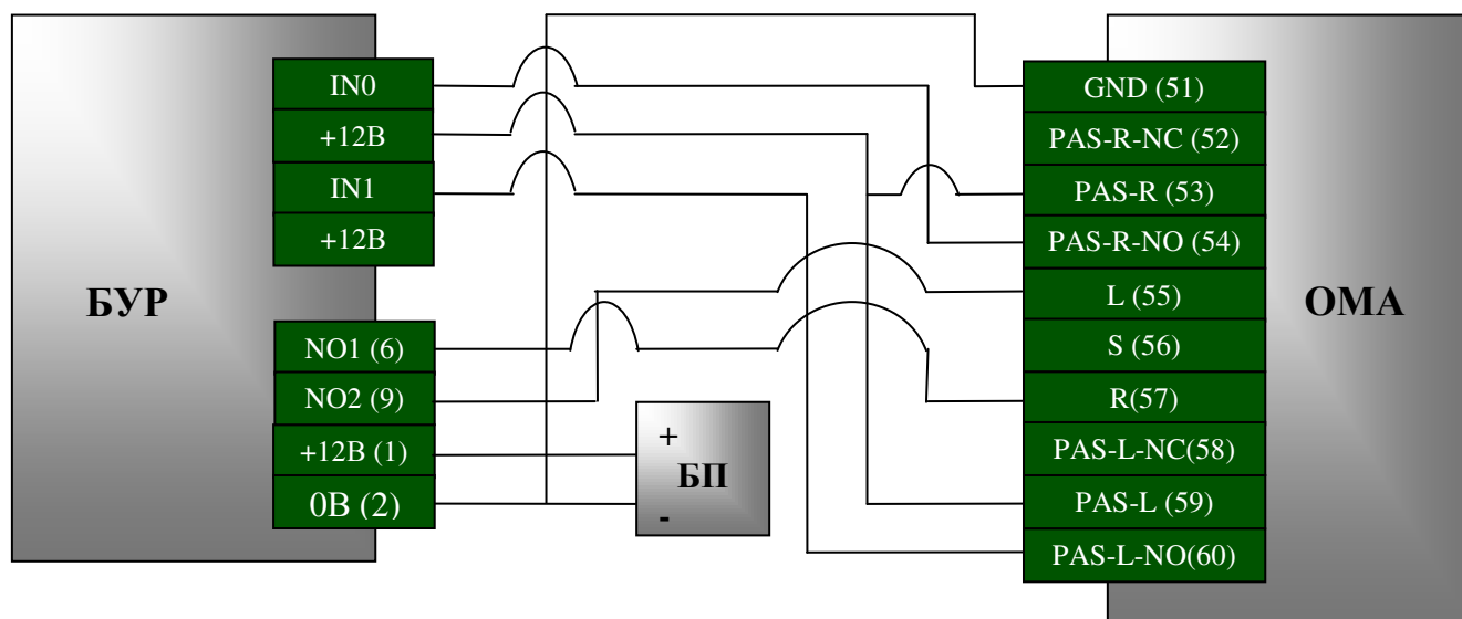
Рисунок 10: Подключение турникета ОМА
