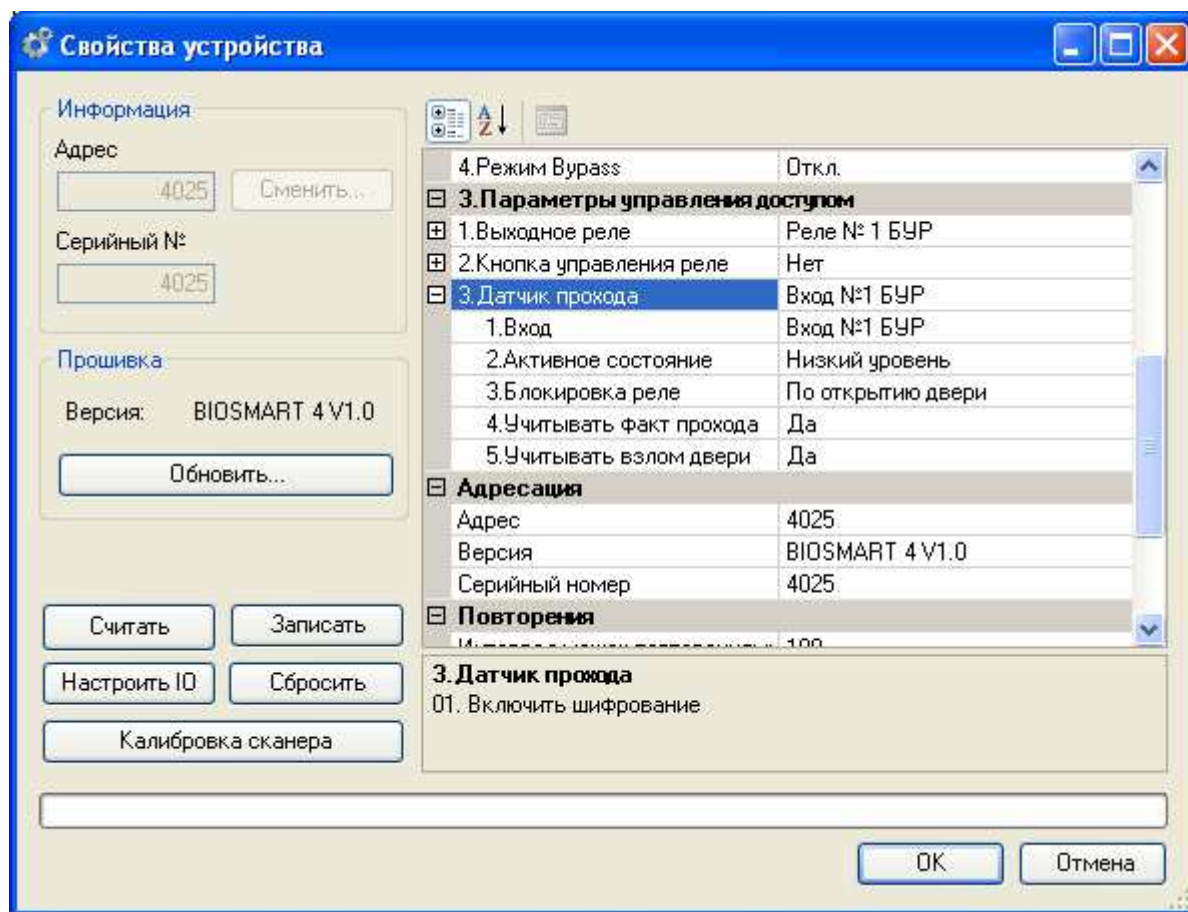
Рисунок 7: Окно настройки датчика двери
