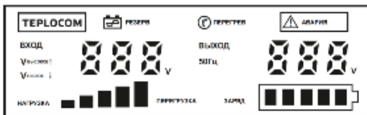
Рисунок 4 — Светодиодный графический индикатор.
