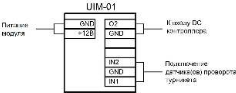
Рисунок 2. Схема платы модуля UIM-01
