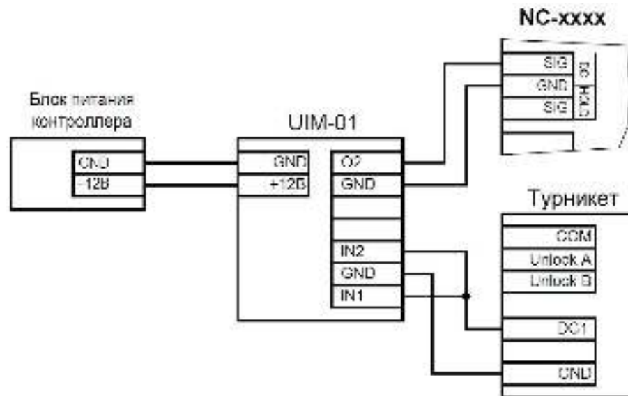
Рисунок 3. Подключение турникета с одним датчиком проворота
