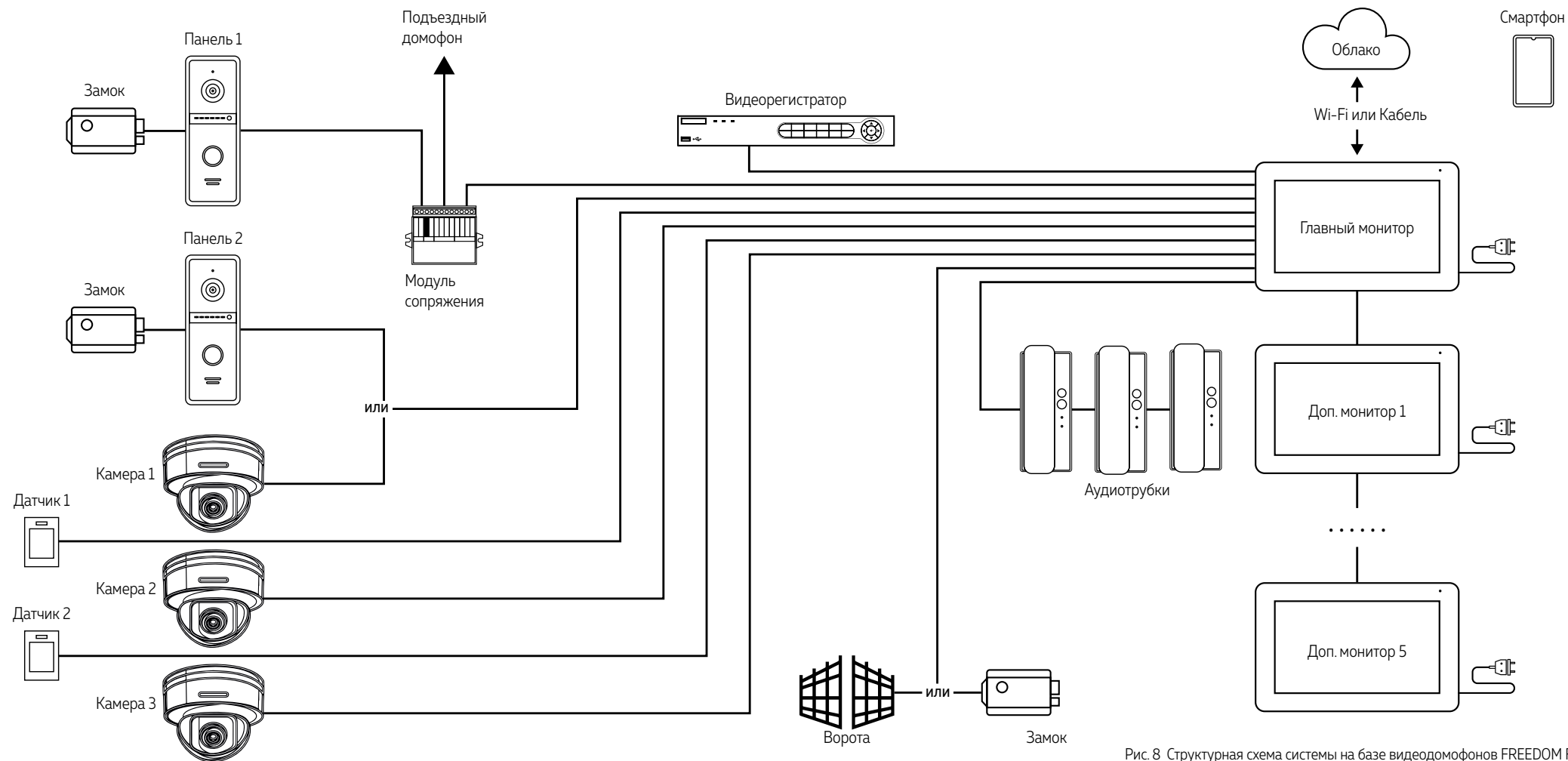
Рис. 8 Структурная схема системы на базе видеодомофонов FREEDOM FHD WIFI
