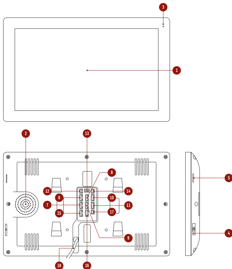
Рис. 3 Описание монитора видеодомофона FREEDOM 10 FHD WIFI
