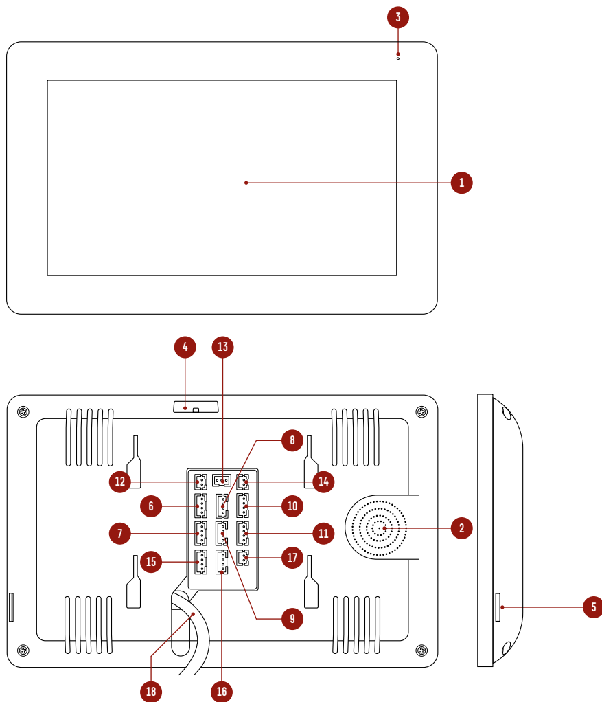
Рис. 2. Описание монитора видеодомофона FREEDOM 7 FHD WIFI
