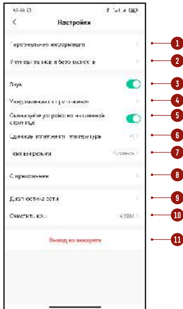
Рис. 77 Настройка Профиля
