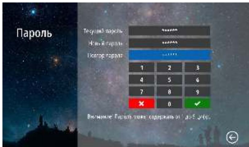
Рис. 41 Изменение мастер-пароля
