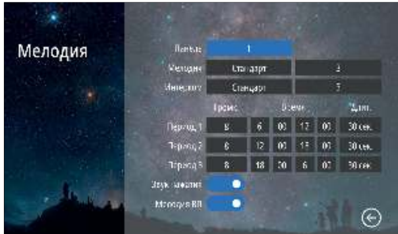
Рис. 34 Подменю "Мелодия"
