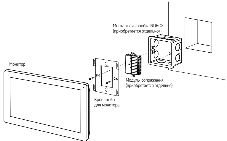
Рис. 5 Монтаж монитора видеодомофона FREEDOM
