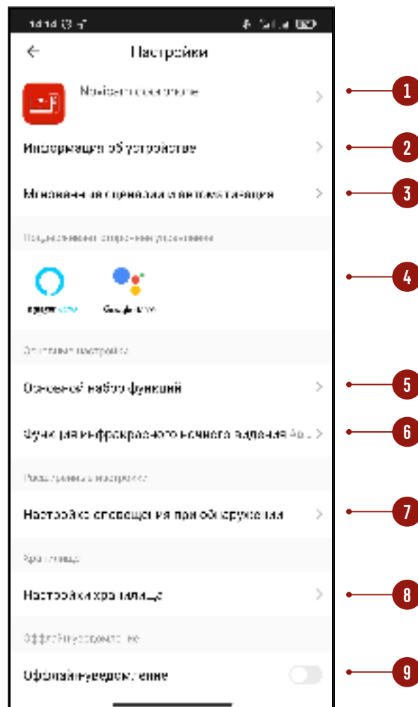
Рис. 74 Меню настроек
