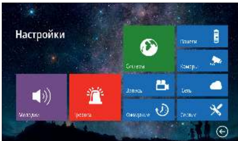
Рис. 30 Меню "Настройки"
