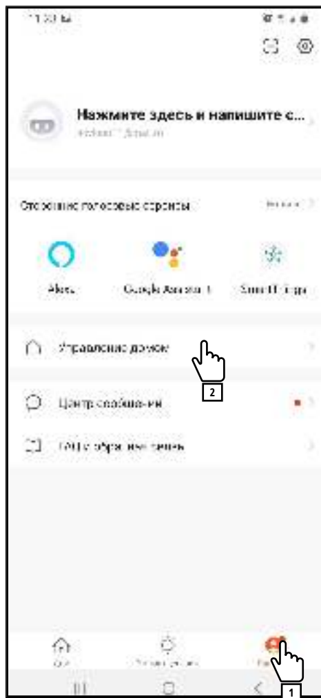
Рис. 78 Управление Домом
