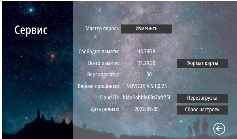
Рис. 40 Подменю "Сервис"
