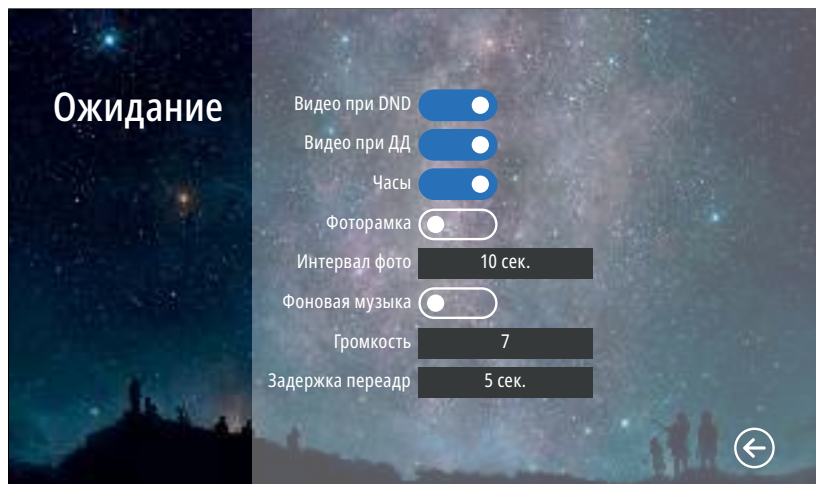
Рис. 37 Подменю "Ожидание"
