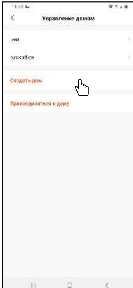
Рис. 79 Создание Дома
