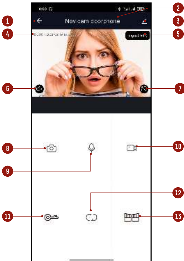
Рис. 71 Меню устройства
