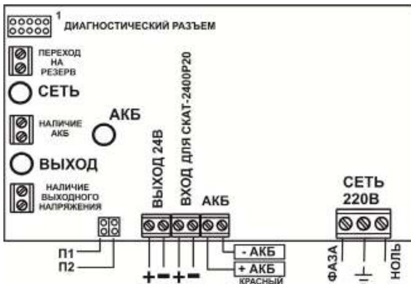
Рисунок 1. Вид источника с открытой крышкой (схема подключения)
