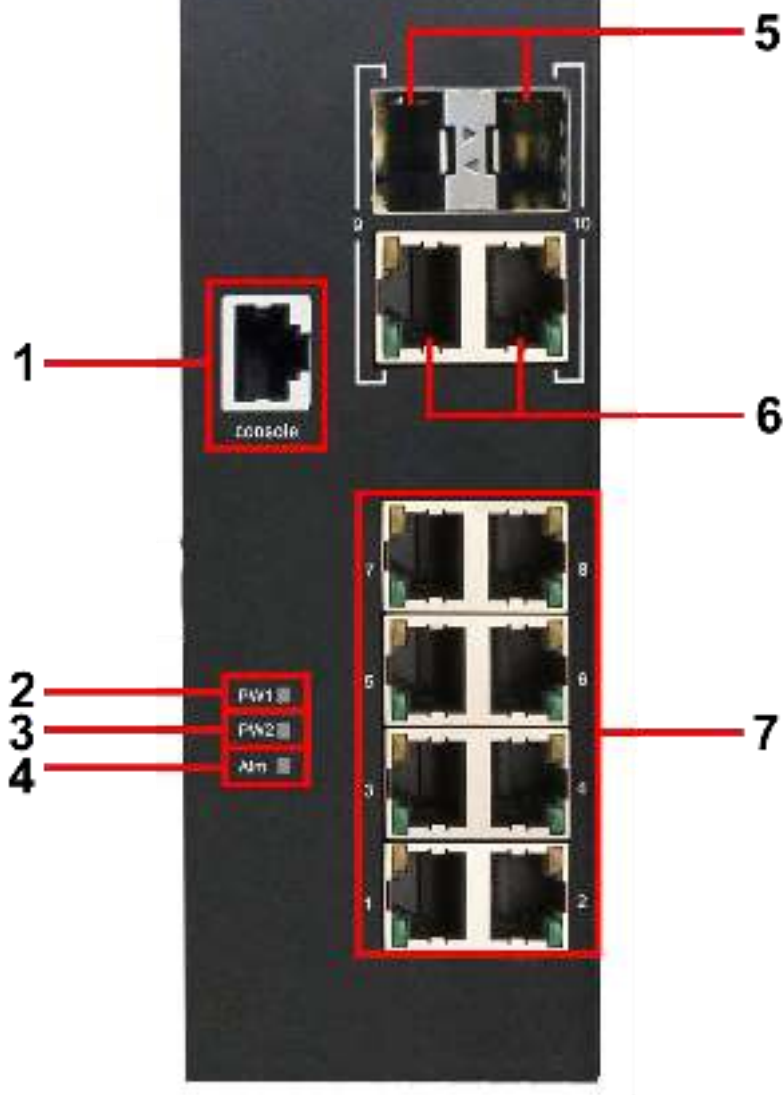
Рис. 2 Коммутаторы SW-60822/ILR(SW-80822/ILR), разъемы, кнопки и индикаторы передней панели
