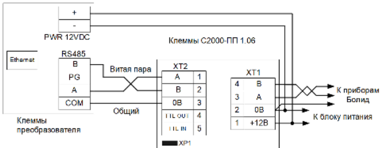
Рис. 1. Схема подключения преобразователя.
