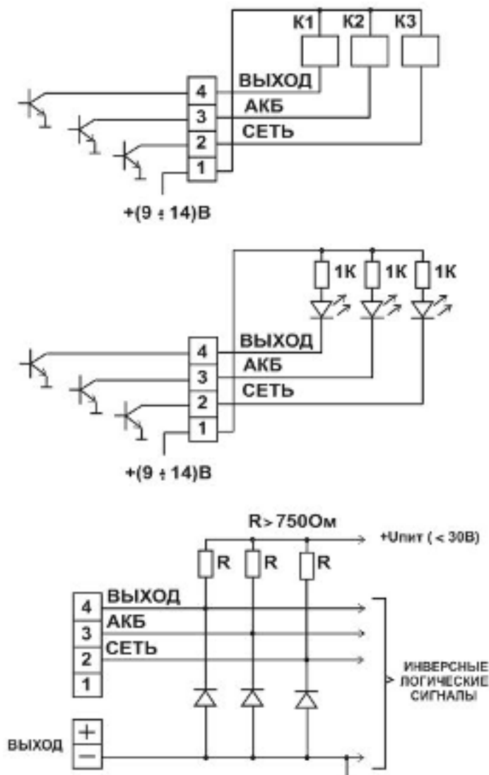
Рисунок 2. Примеры схем подключения исполнительных устройств к выходам «открытый коллектор»
