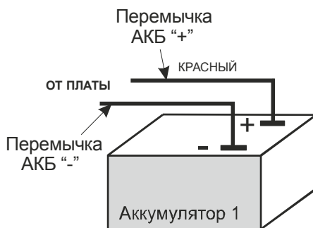
Рисунок 4. Подключение одного аккумулятора
