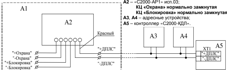
Рисунок 1 Схема соединений
