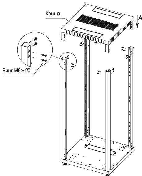
Рисунок 3 – Установка крыши
