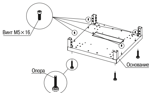
Рисунок 1 – Основание
