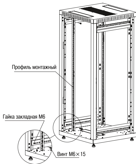
Рисунок 5 – Установка монтажных профилей
