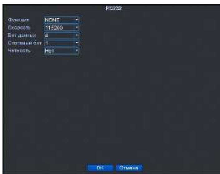
Рисунок 4.34 Настройки последовательного порта
