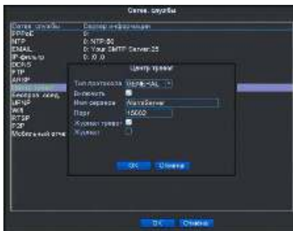
Рисунок 4.25 Настройки сервера Центра тревог
