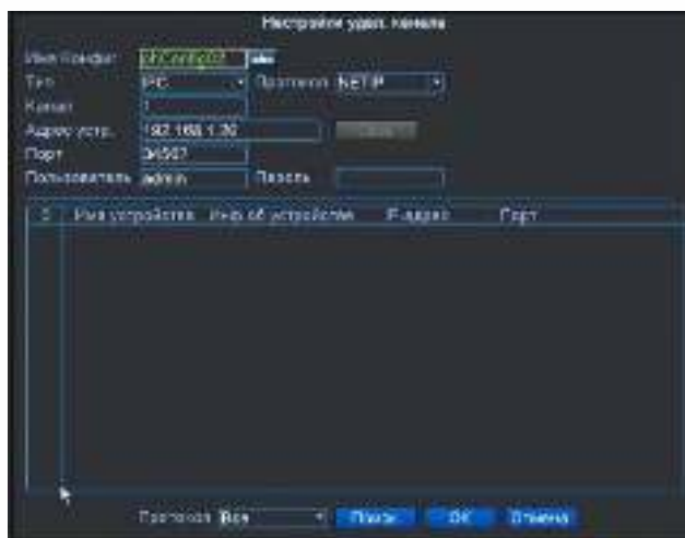
Рисунок 4.38 Страница добавления удаленного устройства.
