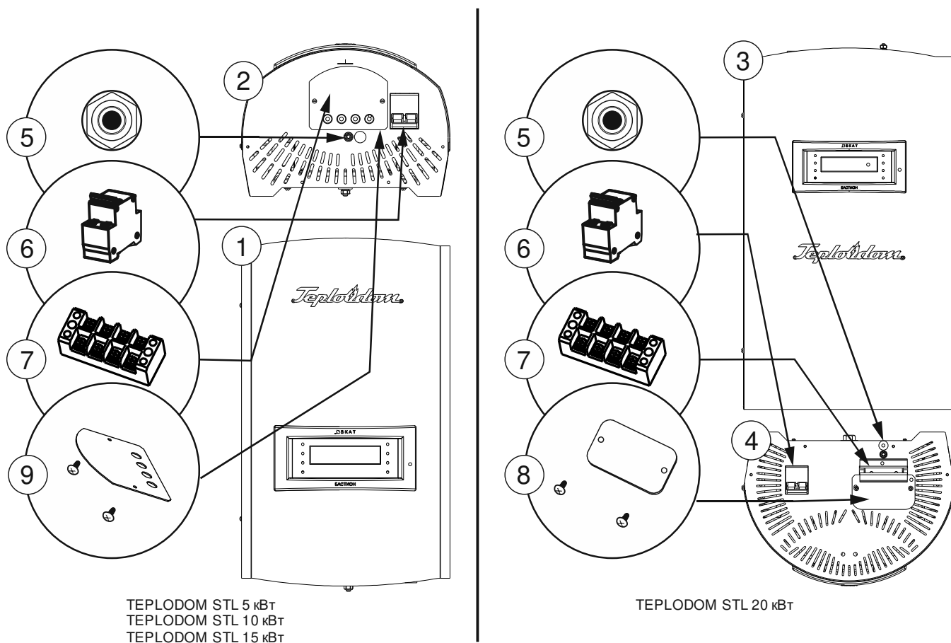
Рисунок 1. Общий вид стабилизатора и его функциональных элементов
