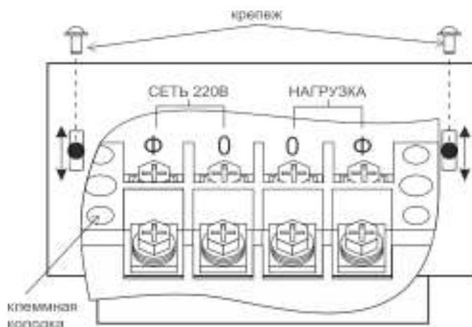
Рисунок 3. Схема подключения к клеммной колодке
