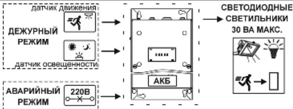
Рисунок 1 – варианты подключения
