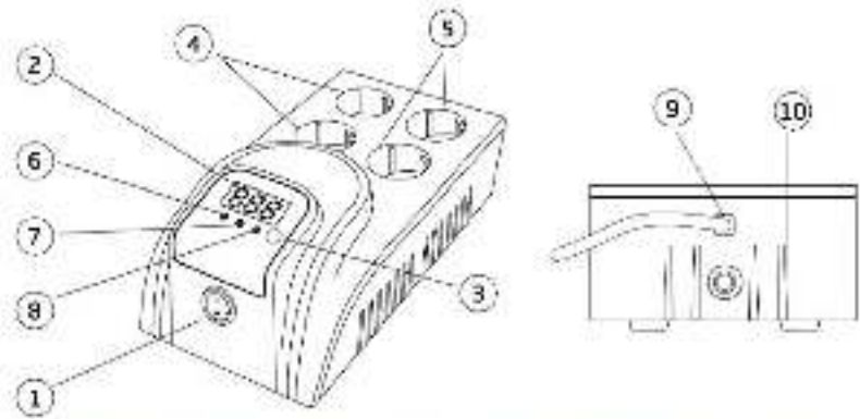
Рисунок 1. Внешний вид стабилизатора напряжения SMARTWATT AVR HOME 500-1000VA. Описание элементов приводится в таблице 1.
