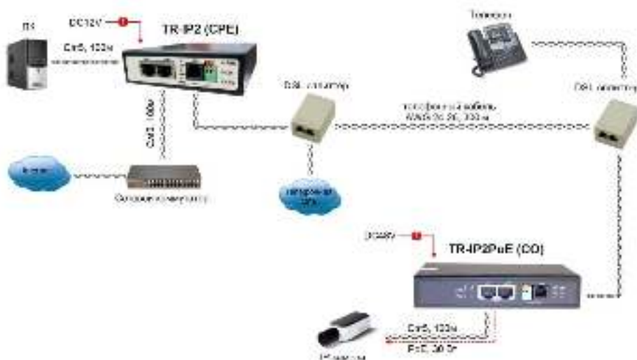
Рис. 7а Схема подключения TR-IP2PoE (CO) и TR-IP2 (CPE) для организации IP-видеонаблюдения с передачей питания на сетевые устройства.
